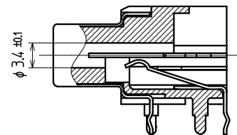
内部構造図
