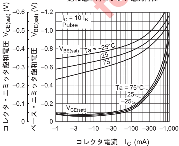
飽和電圧対コレクタ電流特性
