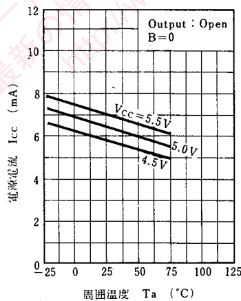
I_{CC} - T_a
