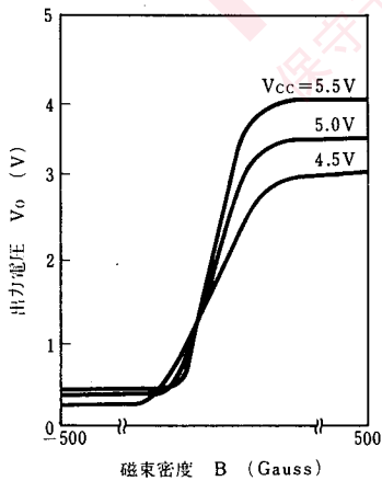
V_O - B
