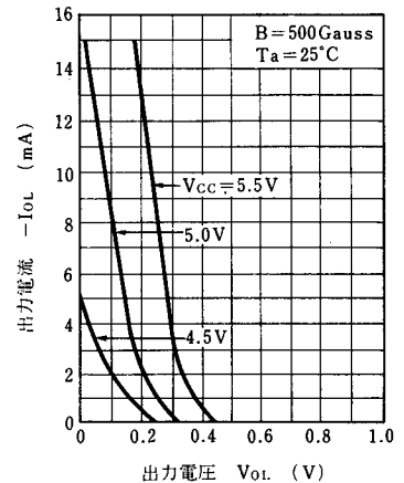
I_{OL} - V_{OL}
